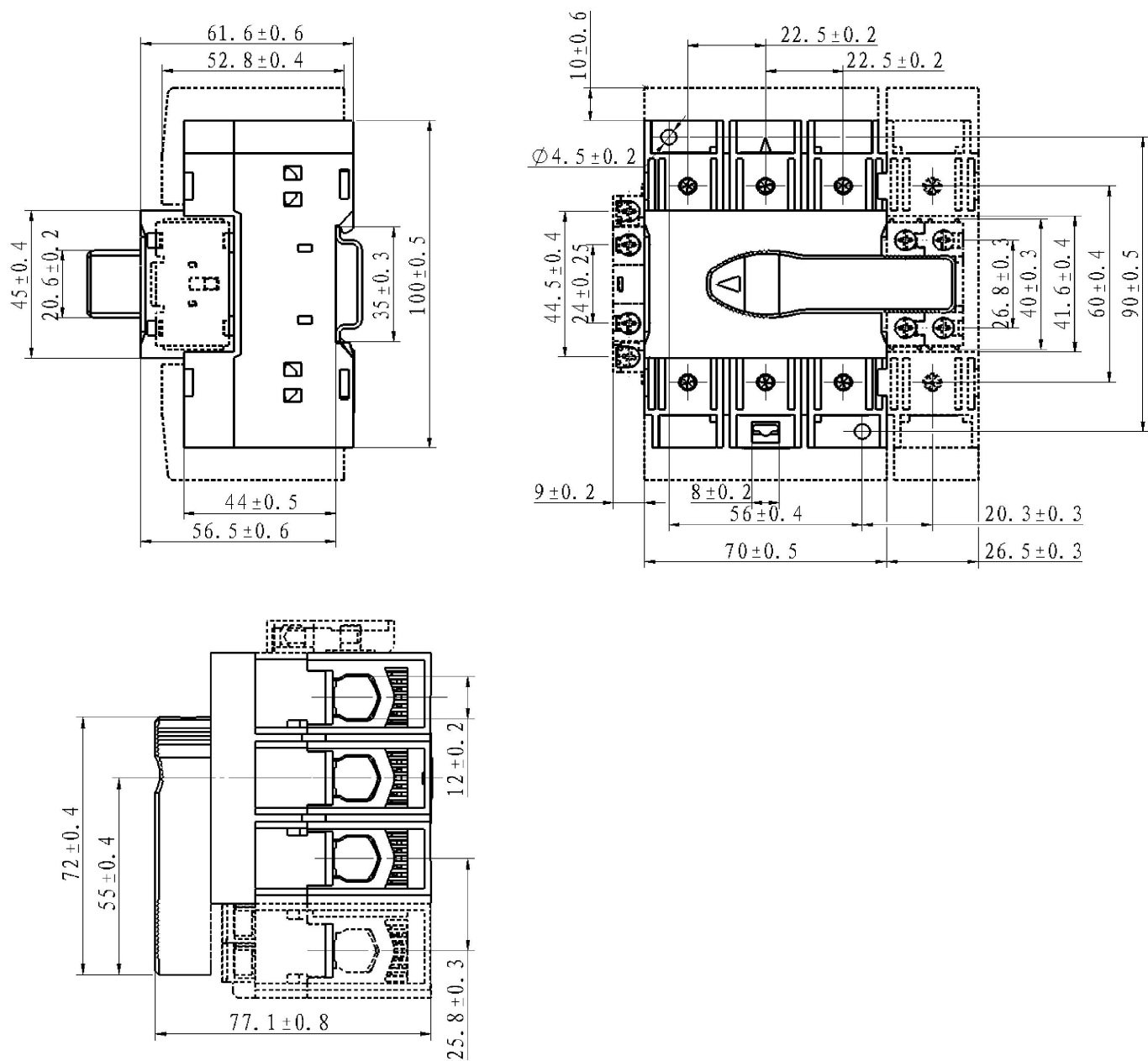
ГАБАРИТНЫЕ РАЗМЕРЫ ВН-IS 125AF стационарная (выносная) рукоятка на корпусе
