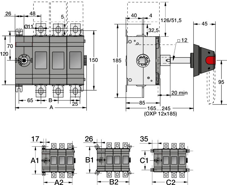
ГАБАРИТНЫЕ РАЗМЕРЫ ВН-IS -D 400А С ПЕРЕДНЕЙ ВЫНОСНОЙ РУКОЯТКОЙ
