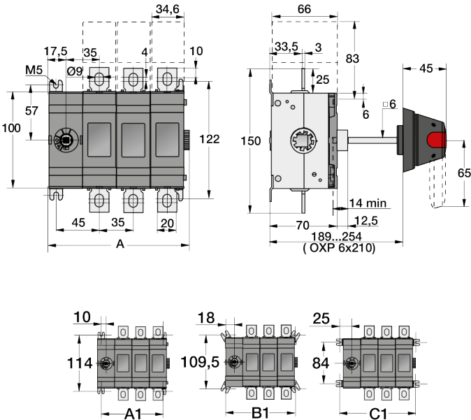
ГАБАРИТНЫЕ РАЗМЕРЫ ВН-IS-D 125А, 160А, 250А С ПЕРЕДНЕЙ ВЫНОСНОЙ РУКОЯТКОЙ
