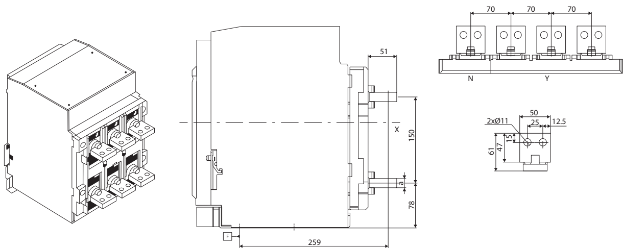
ПРИСОЕДИНИТЕЛЬНЫЕ РАЗМЕРЫ ВAB-C(02~16)-70ВВ
