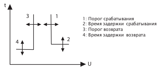
Принцип действия функции защиты от перенапряжения
