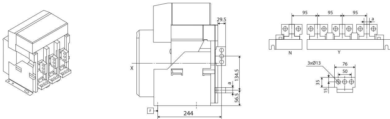
ПРИСОЕДИНИТЕЛЬНЫЕ РАЗМЕРЫ ВАВ-С(20~25)-65(85)СК2
