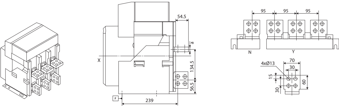
ПРИСОЕДИНИТЕЛЬНЫЕ РАЗМЕРЫ ВAB-C(06~25)-1140-50CK1
