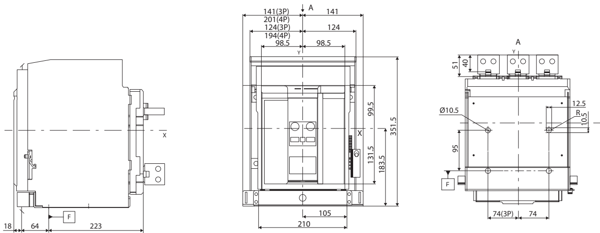
ПРИСОЕДИНИТЕЛЬНЫЕ РАЗМЕРЫ ВAB-C(02~16)-70ВГ
