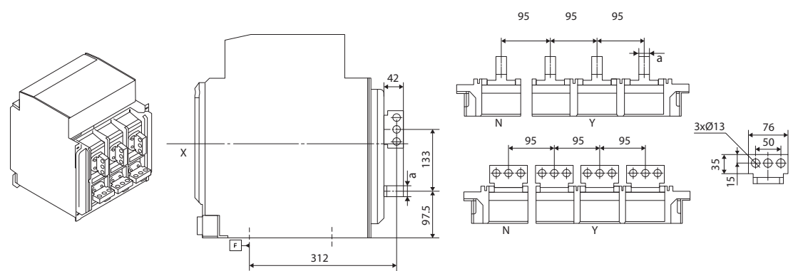
ПРИСОЕДИНИТЕЛЬНЫЕ РАЗМЕРЫ ВAB-C(20~25)-65(85)BK2
