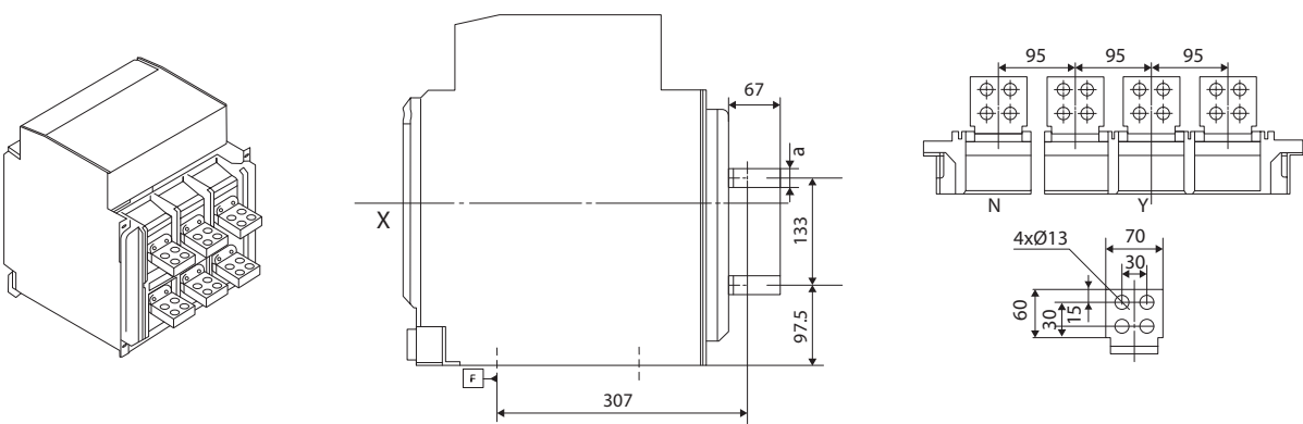
ПРИСОЕДИНИТЕЛЬНЫЕ РАЗМЕРЫ ВAB-C(06~25)-1140-50BB
