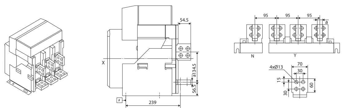
ПРИСОЕДИНИТЕЛЬНЫЕ РАЗМЕРЫ ВAB-C(06~25)-1140-50CK2
