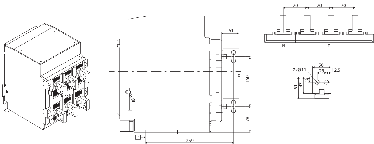
ПРИСОЕДИНИТЕЛЬНЫЕ РАЗМЕРЫ ВAB-C(02~16)-70ВВ
