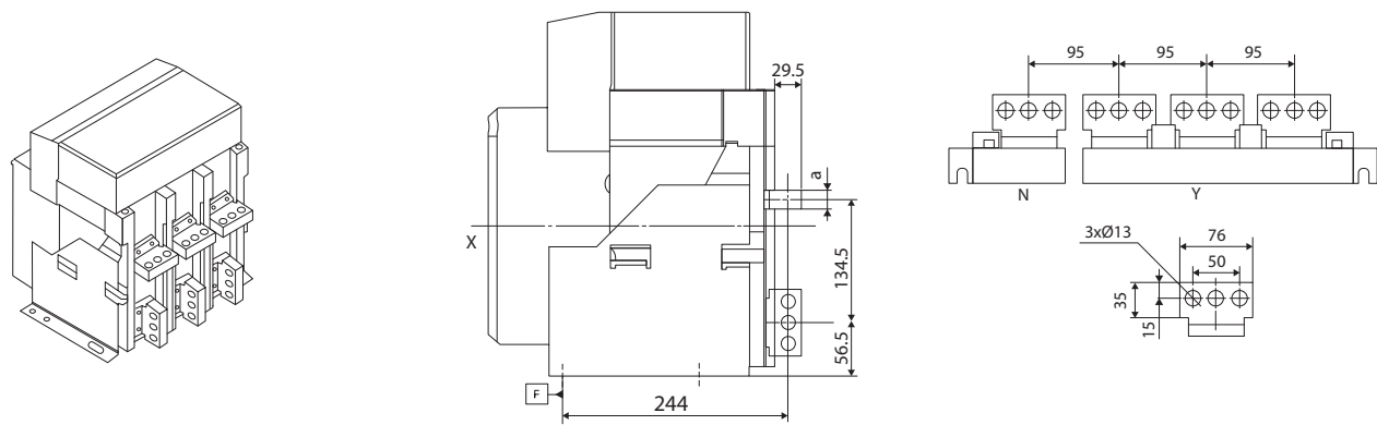
ПРИСОЕДИНИТЕЛЬНЫЕ РАЗМЕРЫ ВАВ-С(20~25)-65(85)СК1
