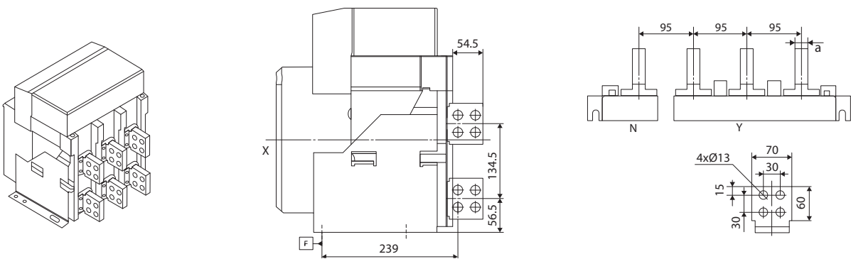
ПРИСОЕДИНИТЕЛЬНЫЕ РАЗМЕРЫ ВAB-C(06~25)-1140-50CB
