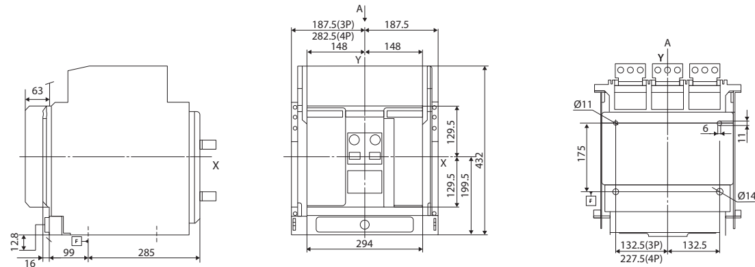
ПРИСОЕДИНИТЕЛЬНЫЕ РАЗМЕРЫ ВАВ-С(20~25)-65(85)ВГ
