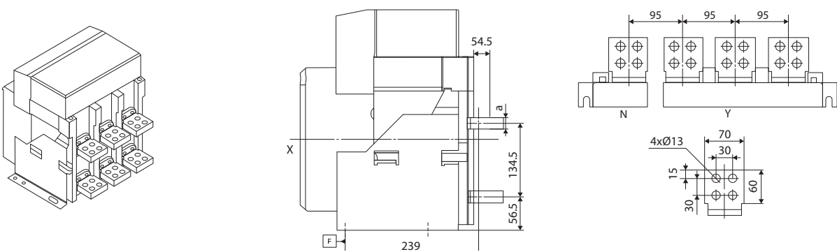
ПРИСОЕДИНИТЕЛЬНЫЕ РАЗМЕРЫ ВAB-C(06~25)-1140-50CГ
