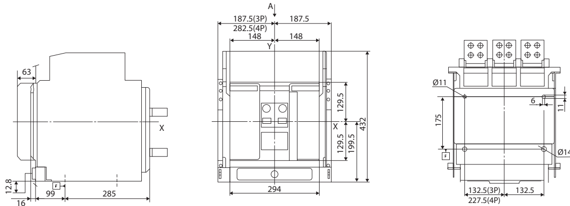
ГАБАРИТНЫЕ И УСТАНОВОЧНЫЕ РАЗМЕРЫ ВAB-C(06~25)-1140-50B (ВЫКАТНОЕ ИСПОЛНЕНИЕ)
