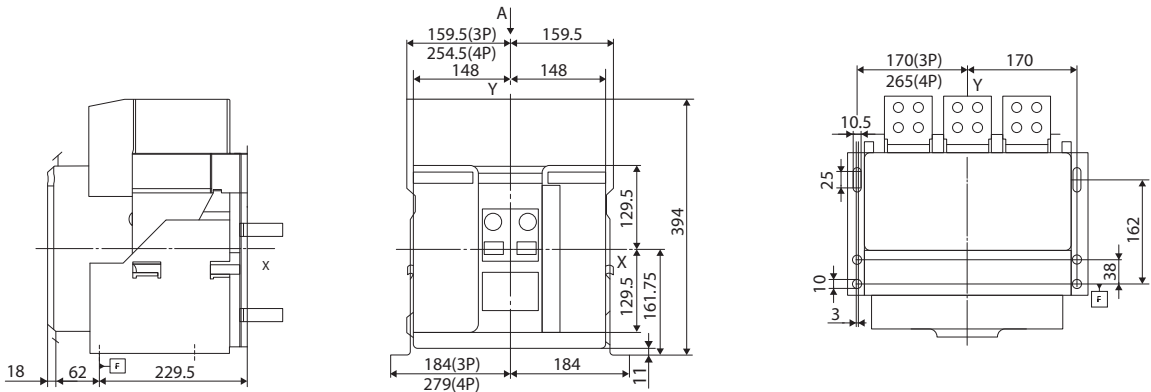
ГАБАРИТНЫЕ И УСТАНОВОЧНЫЕ РАЗМЕРЫ ВAB-C(06~25)-1140-50C (СТАЦИОНАРНОЕ ИСПОЛНЕНИЕ)
