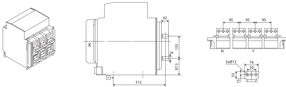
ПРИСОЕДИНИТЕЛЬНЫЕ РАЗМЕРЫ ВАВ-С(20~25)-65(85)ВГ
