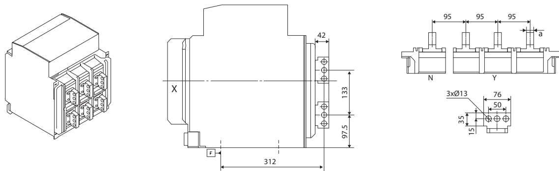
ПРИСОЕДИНИТЕЛЬНЫЕ РАЗМЕРЫ ВАВ-С(20~25)-65(85)ВВ
