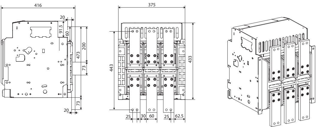
ПРИСОЕДИНИТЕЛЬНЫЕ РАЗМЕРЫ ВAB-C(20~25)-65(85)BП
