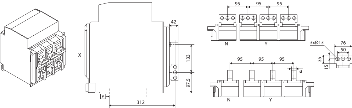
ПРИСОЕДИНИТЕЛЬНЫЕ РАЗМЕРЫ ВAB-C(20~25)-65(85)BK2
