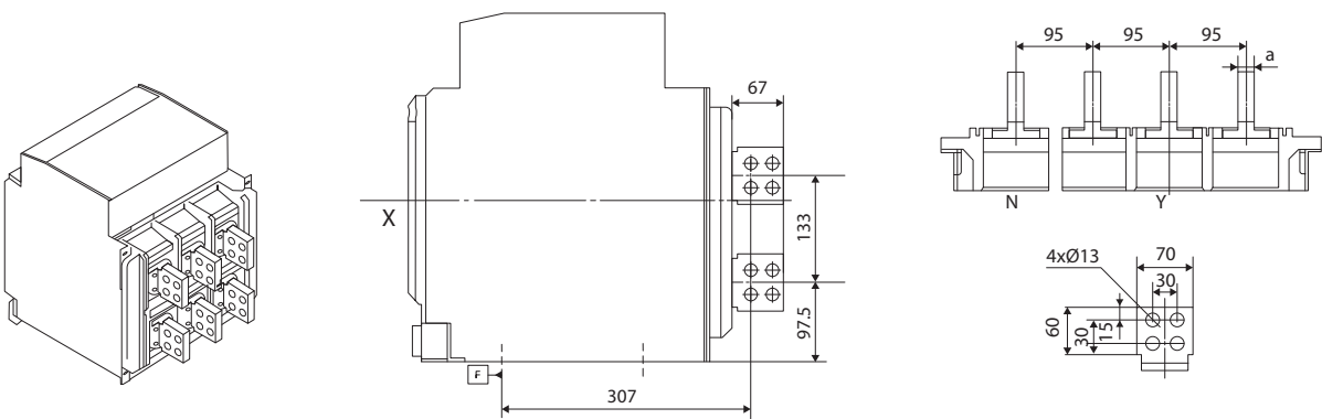
ПРИСОЕДИНИТЕЛЬНЫЕ РАЗМЕРЫ ВAB-C(06~25)-1140-50BB
