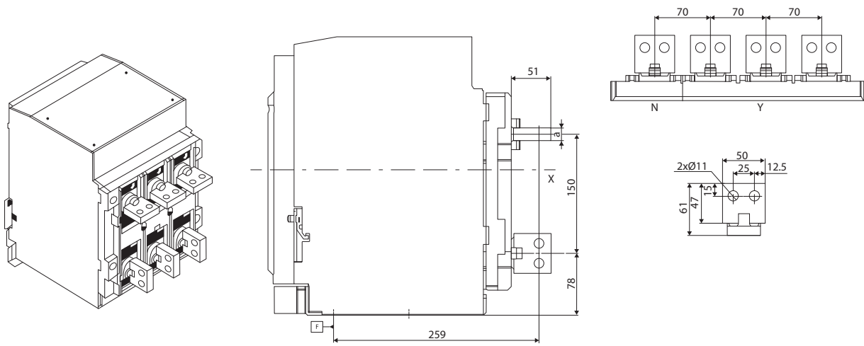
ПРИСОЕДИНИТЕЛЬНЫЕ РАЗМЕРЫ ВAB-C(02~16)-70ВК2
