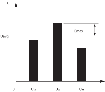
Коэффициент несимметрии напряжений
