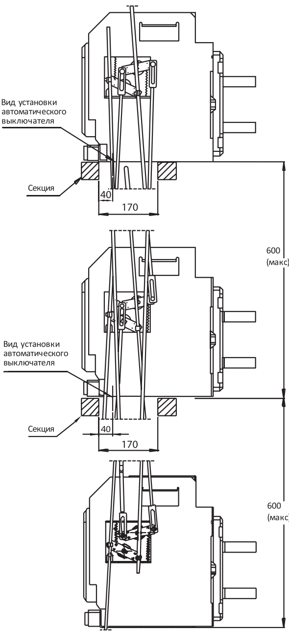
Автоматический выключатель 1
