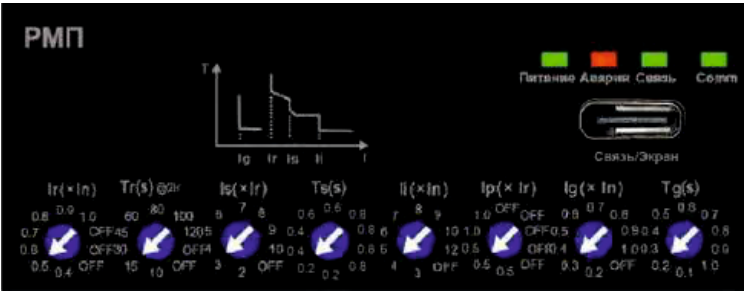
Пример расцепителя РМП
