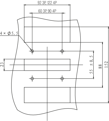
BA57 Aksol 125AF/160AF
