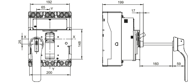
Чертеж габаритных размеров РПВ1600AF-Aksol
