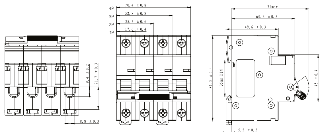
BA47-MCB-L-AKSOL(AC) 15 кА
