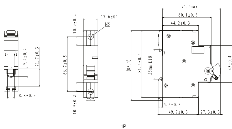
BA47-MCB-L-AKSOL(AC) 15 кА
