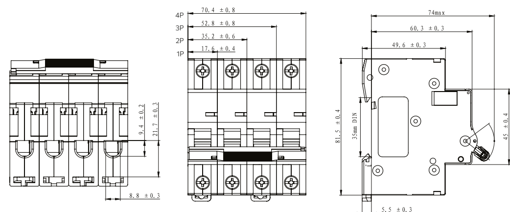
BA47-MCB-N-AKSOL(AC) 10 кА
