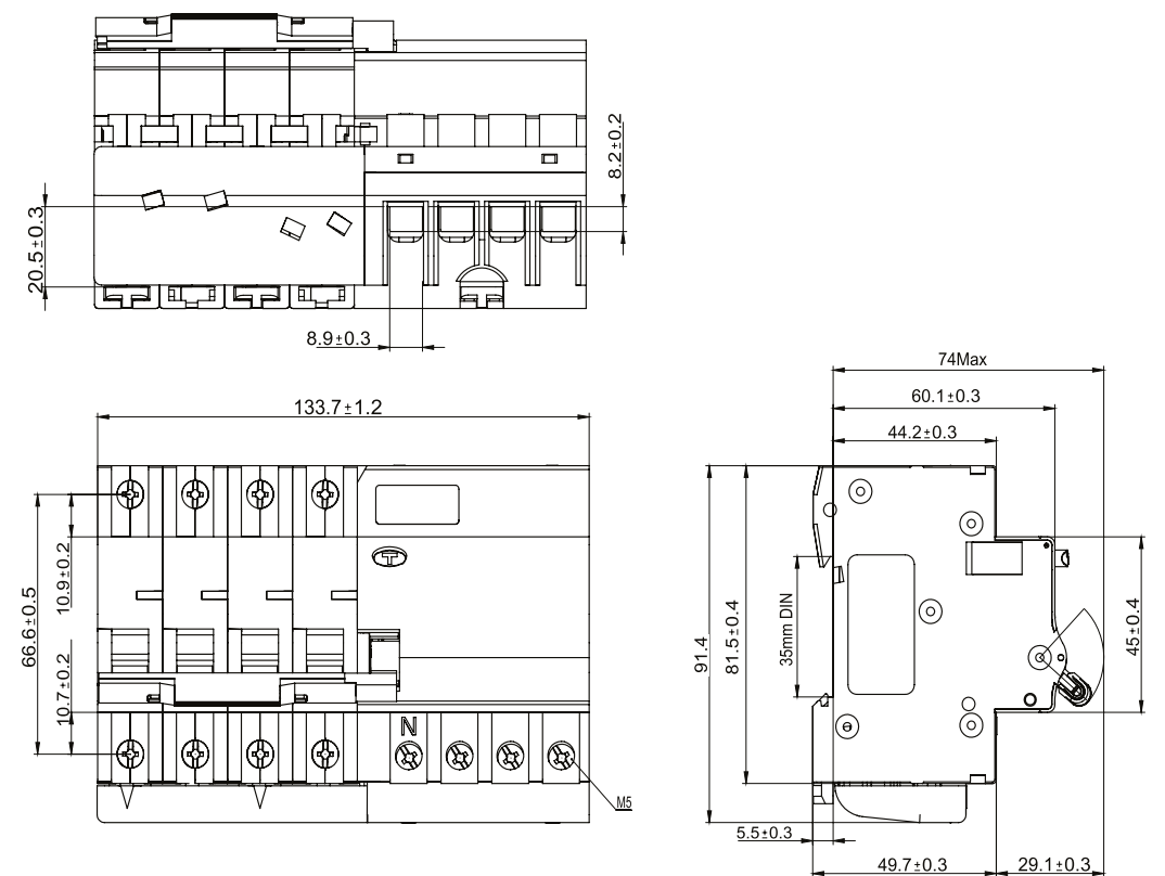
УДТ(М) 4P
