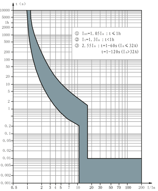
Тип K кривая Защита цепей с преобладающей индуктивной нагрузкой. Мгновенный диапазон срабатывания 9.6-14.4In
