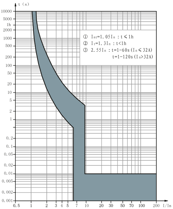
Тип С кривая Защита от обычной нагрузки и распределительного кабеля. Мгновенный диапазон срабатывания 8 (1 ± 20%)
