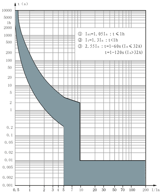
Тип C кривая Защита от обычной нагрузки и распределительного кабеля. Мгновенный диапазон срабатывания 5-10In
