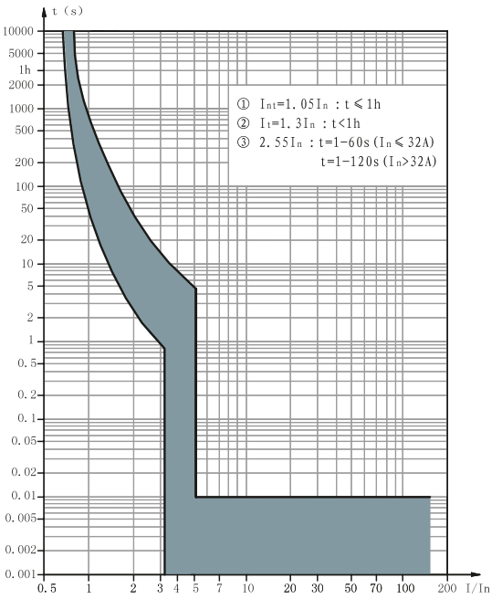
Тип Z кривая Защита цепей с приборами, чувствительными к сверхтокам. Мгновенный диапазон срабатывания 3.2-4.8 In
