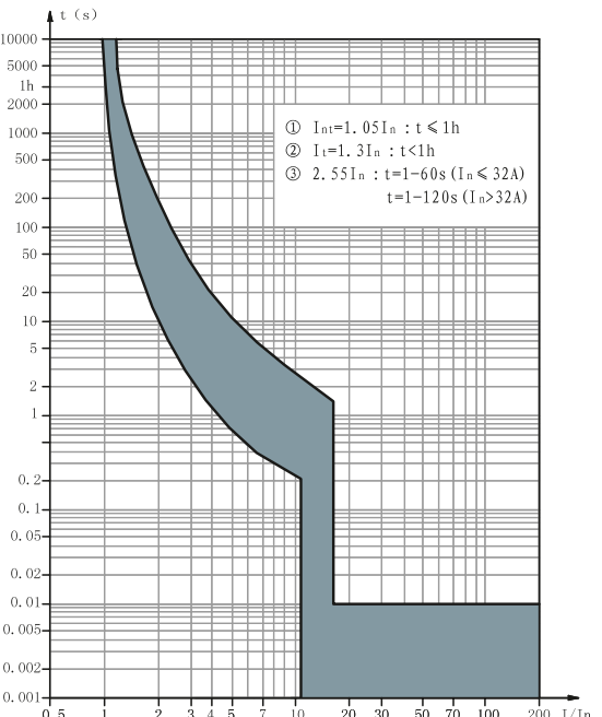
Тип К кривая Защита цепей с преобладающей индуктивной нагрузкой. Мгновенный диапазон срабатывания 14(1±20%)In
