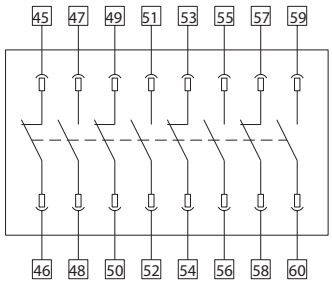
Пять нормально разомкнутых и пять нормально замкнутых
