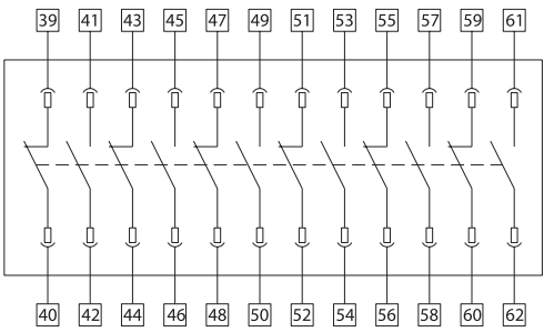
Шесть нормально разомкнутых и шесть нормально замкнутых
