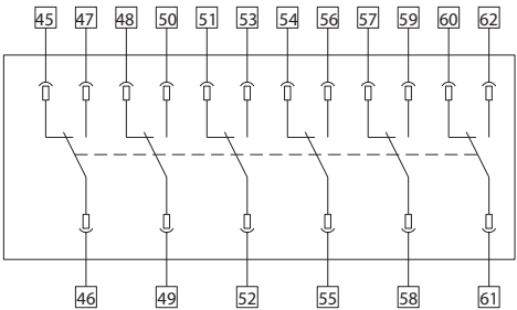
Шесть нормально разомкнутых и шесть нормально замкнутых
