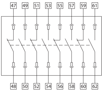
Четыре нормально разомкнутых и четыре нормально замкнутых
