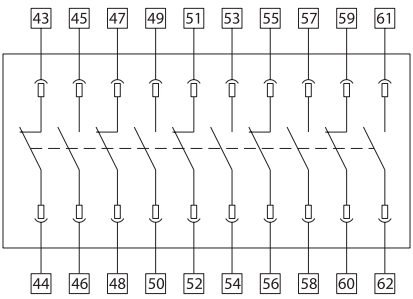
Пять нормально разомкнутых и пять нормально замкнутых
