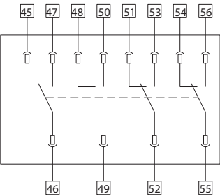
Четыре нормально разомкнутых и четыре нормально замкнутых
