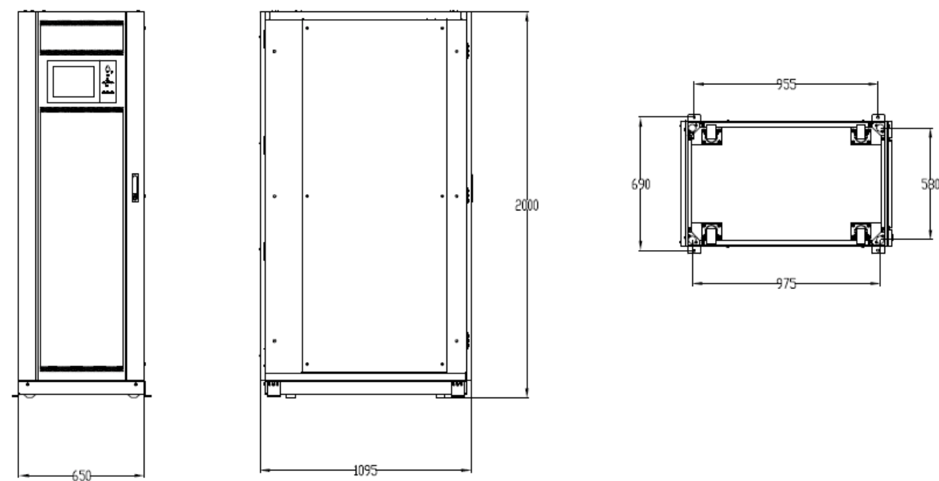
M7B-50050MX*-500 кВА
