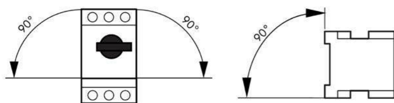
Монтажное положение
