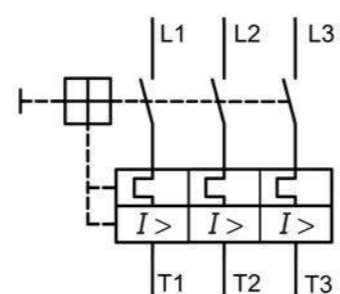
Электрическая схема
