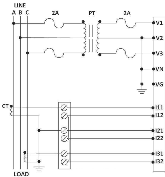
3P 3W 2CT PT
