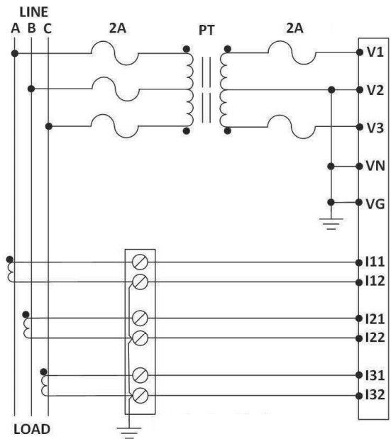
3P 3W 3CT PT
