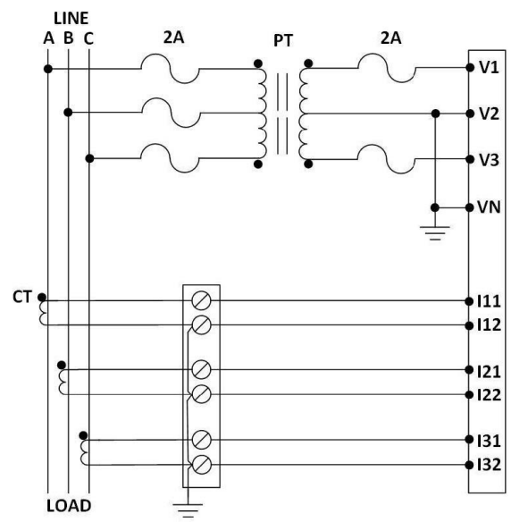
3P 3W 3CT PT
