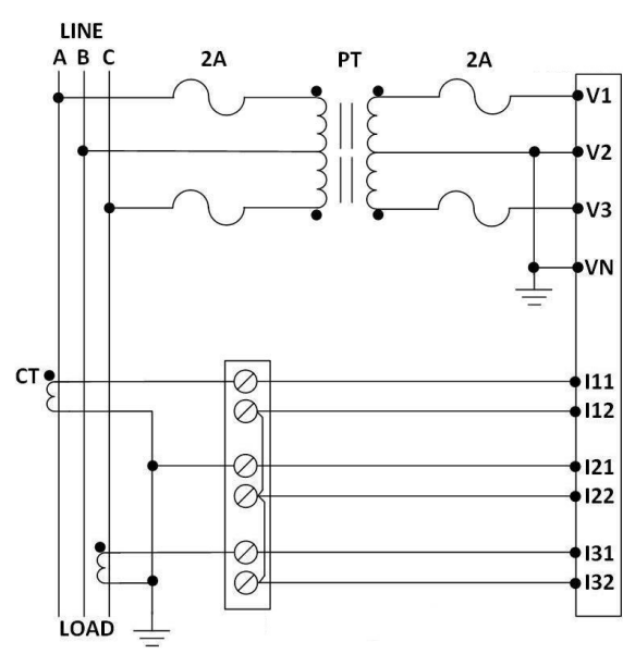
3P 3W 2CT PT
