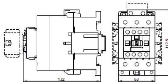
BA47 MC-40-65D (катушка управления AC/DC)
