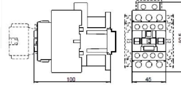
BA47 MC-25-38D (катушка управления AC)
