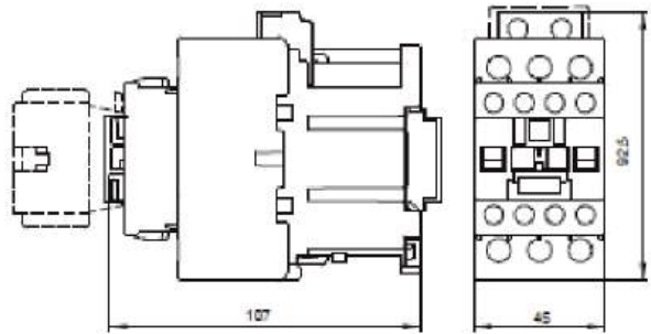
BA47 MC-25-38D (катушка управления DC)
