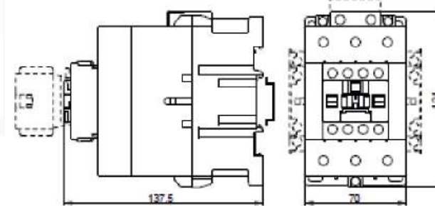
BA47 MC-80-95D (катушка управления AC/DC)
