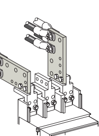
Переднее подключение стационарное исполнение с использованием КПК 1600AF
