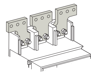
Переднее подключение стационарное исполнение с ПР 1600AF
