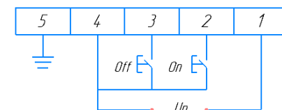
Стандартная схема управления моторным приводом МП BA55-PRO 250AF/630AF NEW
