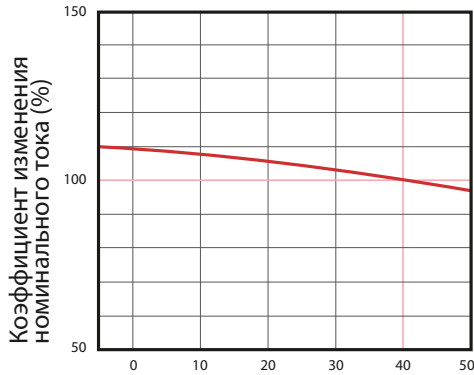
Температура окружающей среды (40°С)
