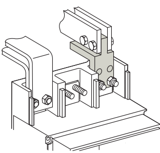
Подключение с ПВП 1600А и без них на стационарном аппарате (выводы переднего подключения)
