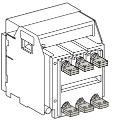
ВБ53-ГГ (питание – горизонтальные, нагрузка – горизонтальные)
