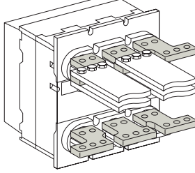
Заднее подключение стационарное исполнение с ПР 1600AF
