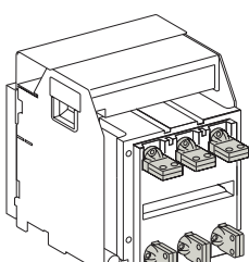
ВБ53-ГВ (питание – горизонтальные, нагрузка – вертикальные)
