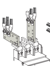
Переднее подключение стационарное исполнение с использованием КПК 1600AF
