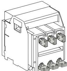
ВБ53-ВГ (питание – вертикальные, нагрузка – горизонтальные)
