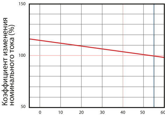
Температура окружающей среды (55°С)
