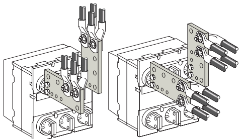
Заднее подключение стационарное исполнение с использованием КПК 1600AF
