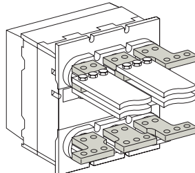
Заднее подключение стационарное исполнение с ПР 1600AF
