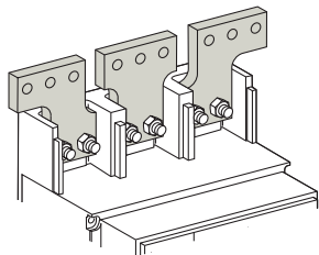
Переднее подключение стационарное исполнение с ПР 1600AF
