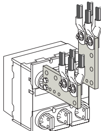
Заднее подключение стационарное исполнение с использованием КПК 1600AF
