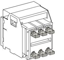
B553-ГГ (питание – горизонтальные, нагрузка – горизонтальные)
